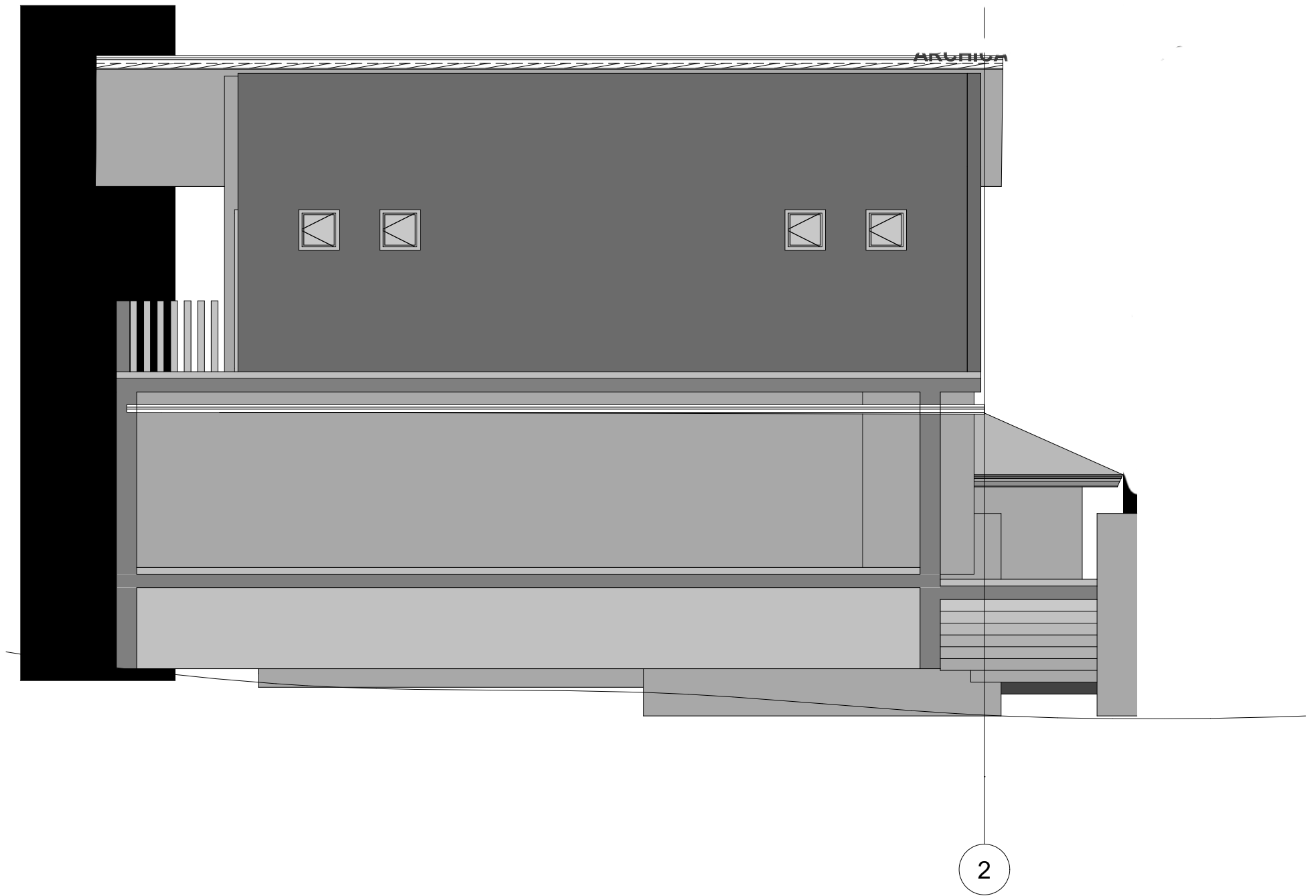
Alzado Oeste
