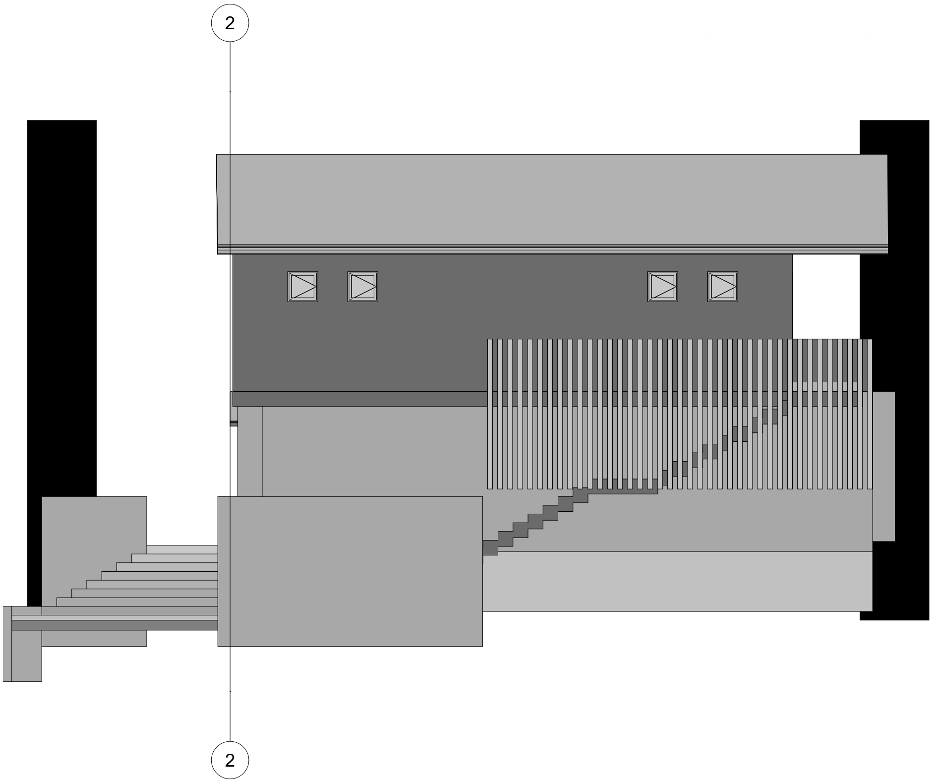
Alzado Este
